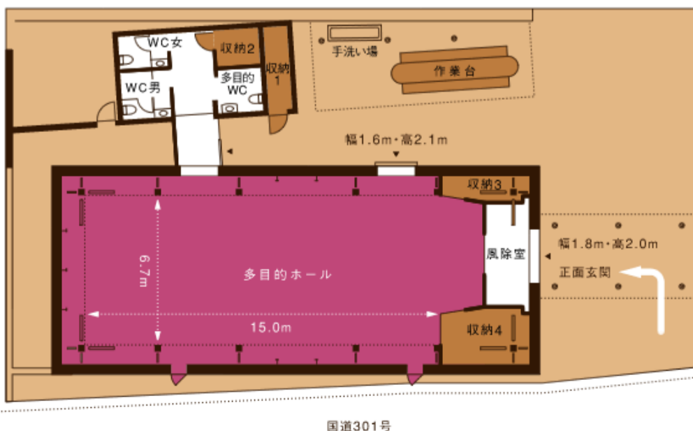
浜名湖れんが館 平面図
